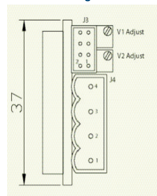
J4Connector : Camden 9200/4A Würth Elektronik 691 352 710 004
